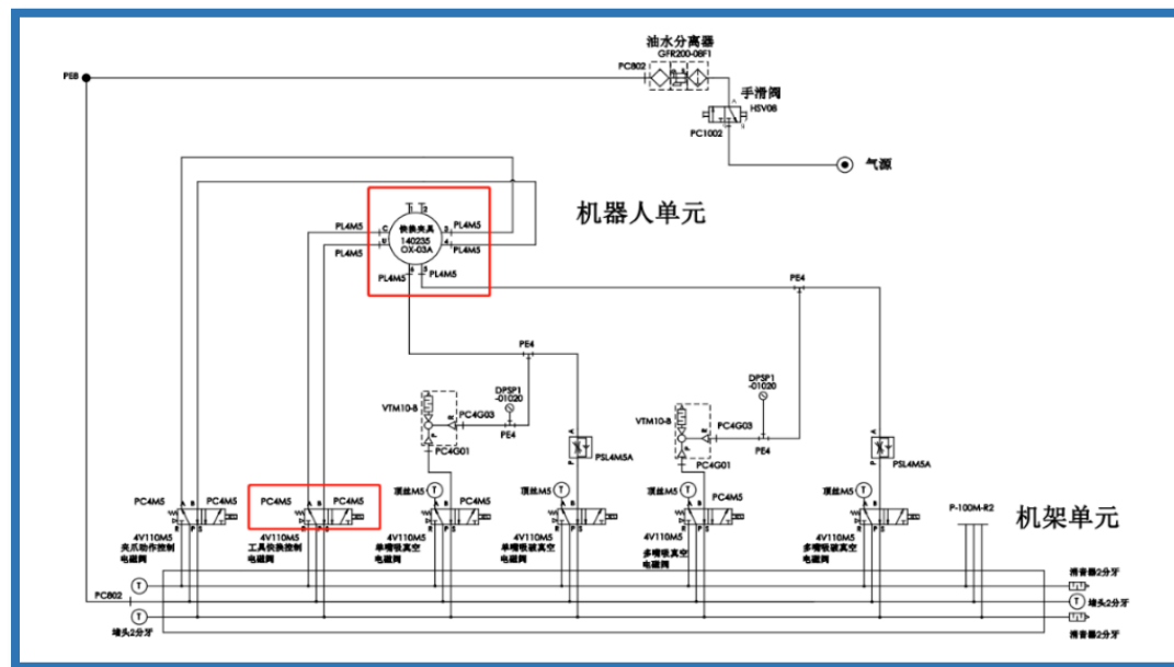
工作站气路图
