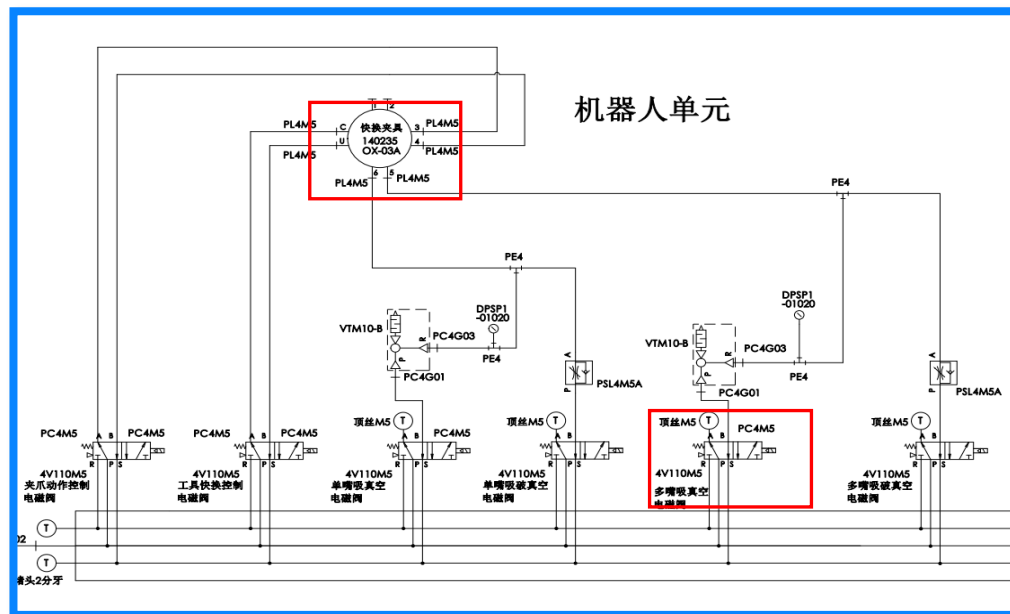
工作站气路图
