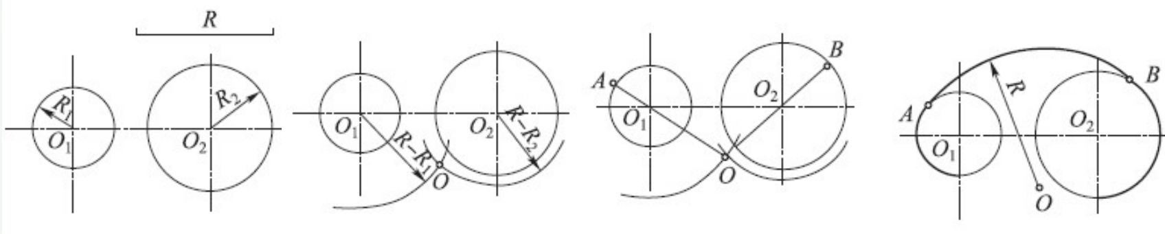
求圆心
