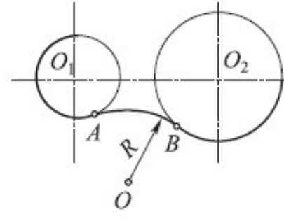
画连接弧
