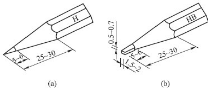
图 1-14 铅笔磨削形状
