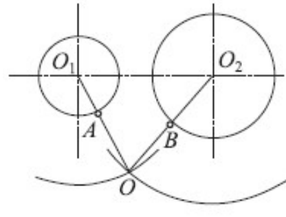
求切点
