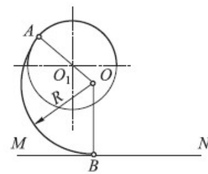
画连接弧
