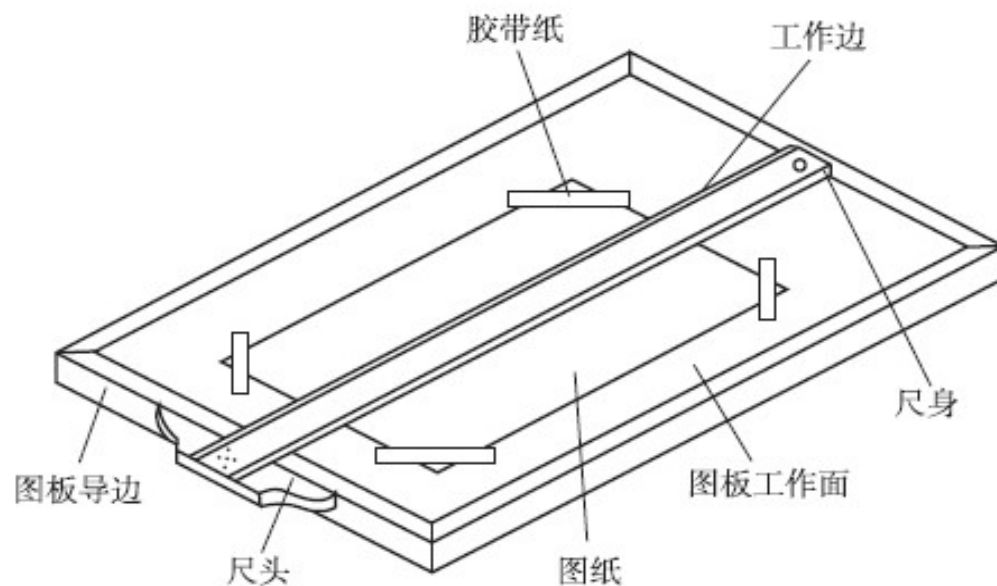
图 1-9 图板和丁字尺
