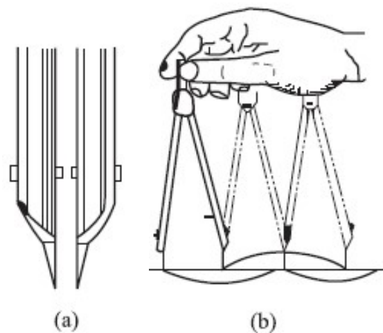
图 1-16 分轨的使用
