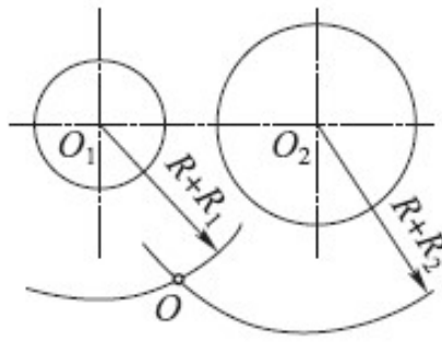
求圆心
